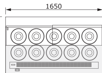
10 POZZETTI CON RISERVA
