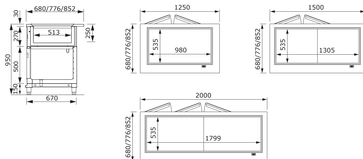
CON CELLA DI RISERVA - WITH STORAGE CELL
