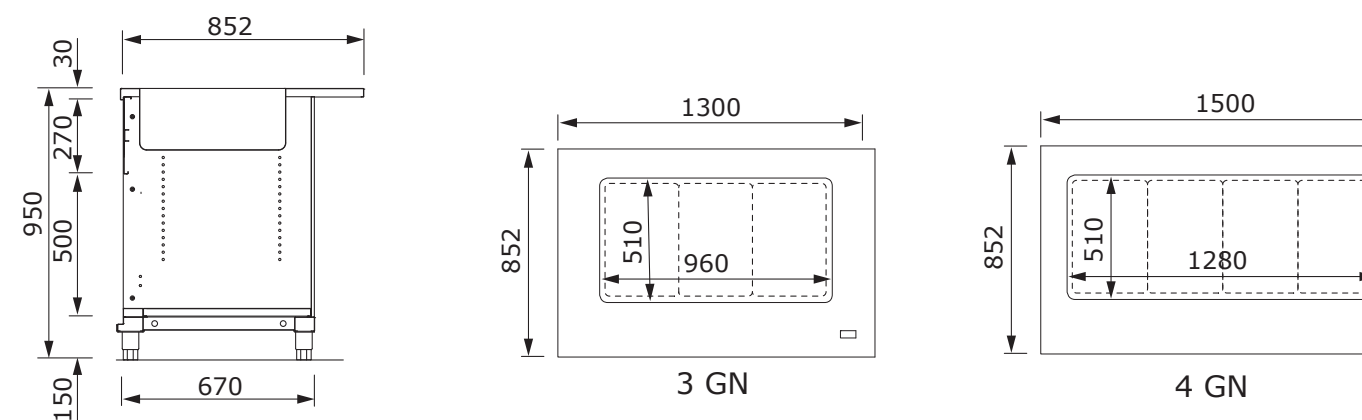
BAGNOMARIA BAIN-MARIE UNIT SU RICHIESTA ON REQUEST
