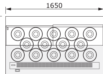
14 POZZETTI CON RISERVA
