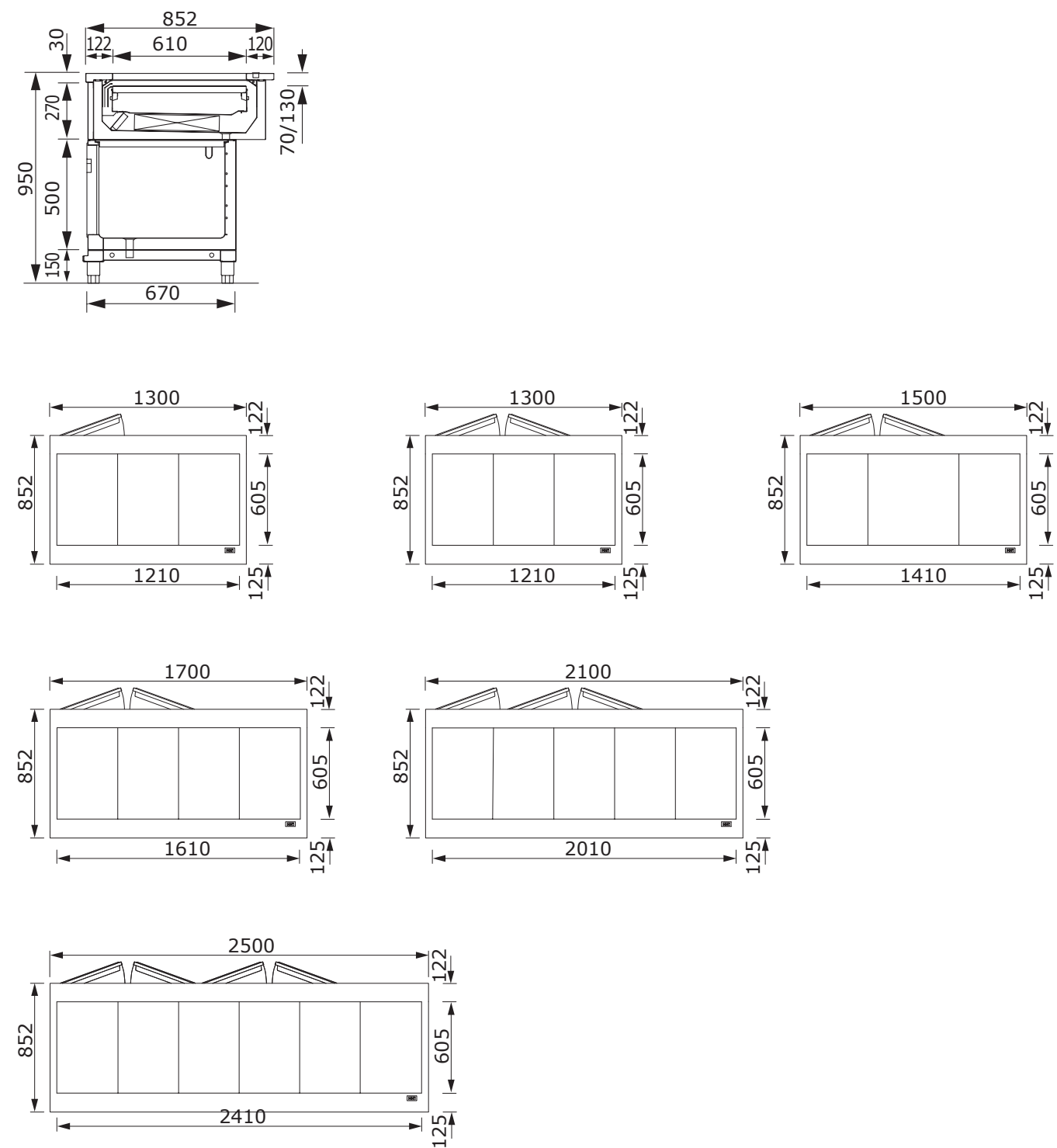
BAGNOMARIA BAIN-MARIE UNIT SU RICHIESTA ON REQUEST
