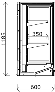
SEZIONE / SIDE VIEWS
