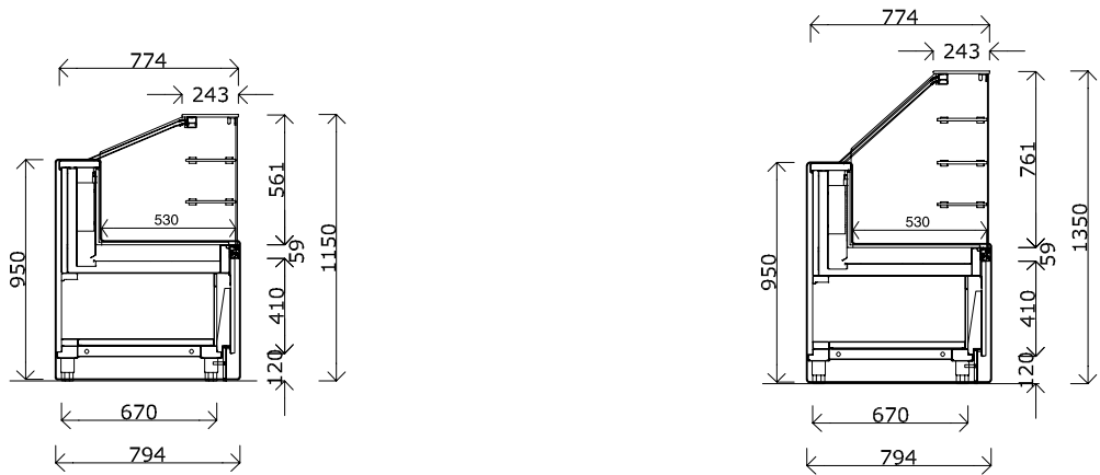
SEZIONI / SIDE VIEWS
