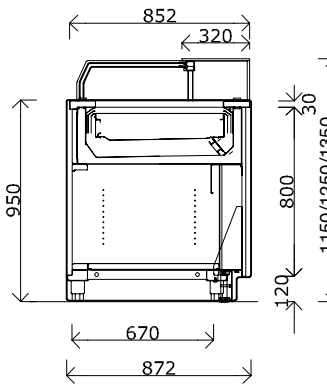
SEZIONI / SIDE VIEWS
