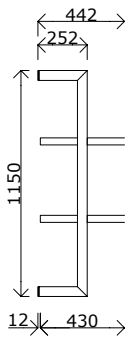
SEZIONE / SIDE VIEW
