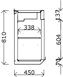
SEZIONE / SIDE VIEWS
