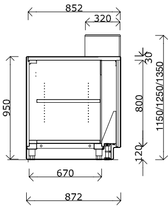
SEZIONI / SIDE VIEWS
