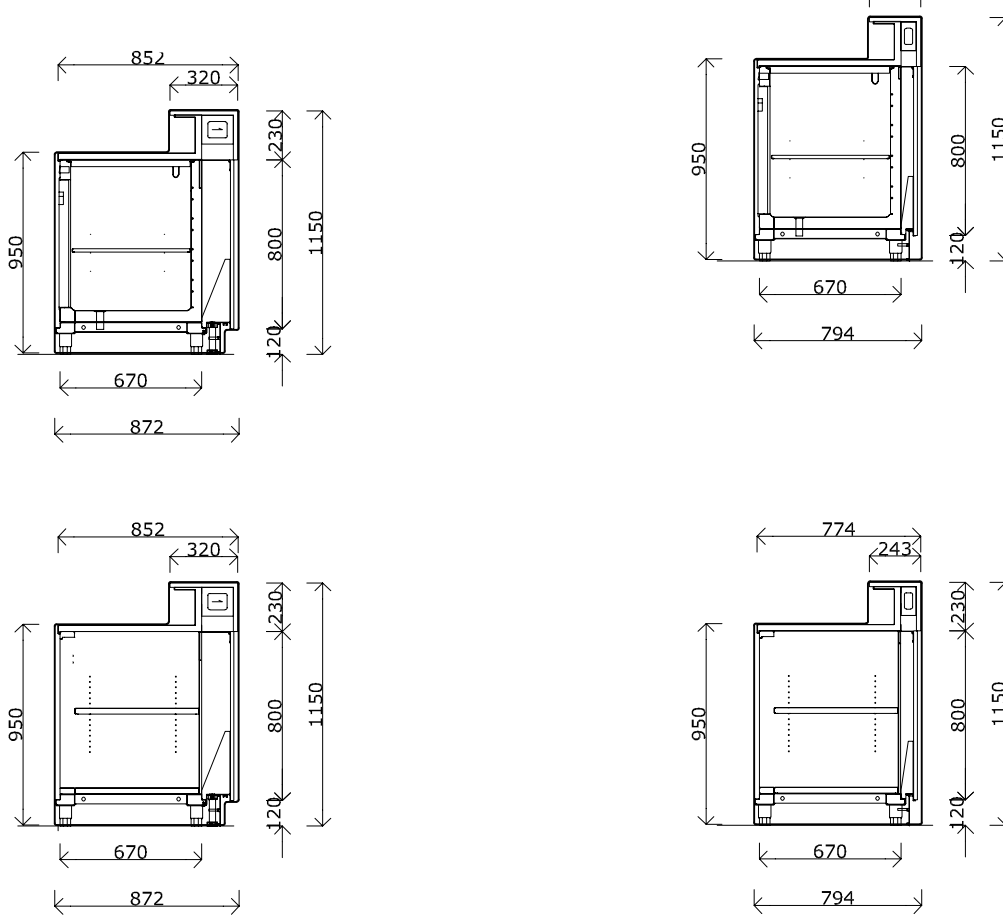
SEZIONI / SIDE VIEWS
