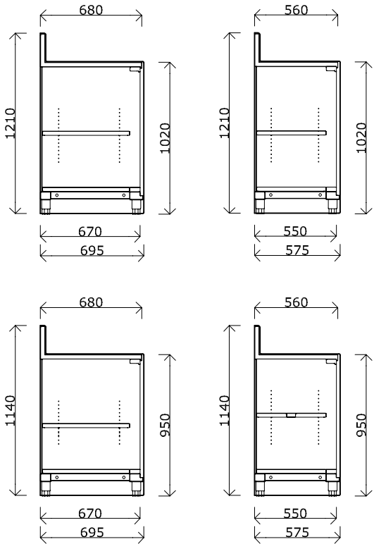
SEZIONE / SIDE VIEWS
