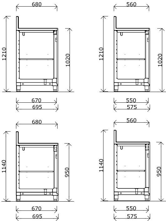
SEZIONI / SIDE VIEWS
