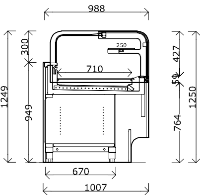
SEZIONI / SIDE VIEWS
