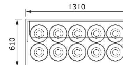
10 POZZETTI CON RISERVA
