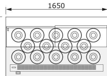
14 POZZETTI CON RISERVA
